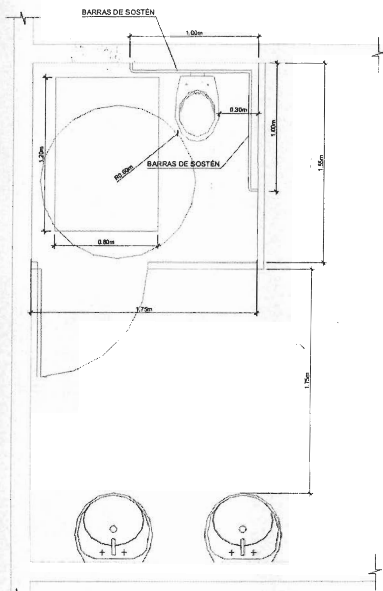
FIGURA 20 DISTRIBUCIÓN EN BAÑOS PÚBLICOS. DIMENSIONES MÍNIMAS DE LOS RECINTOS SANITARIOS UTILIZABLES POR PERSONAS EN SILLAS DE RUEDAS
