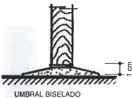
FIGURA 14 UMBRALES DE PUERTAS
